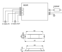
Caractéristiques Philips HID-PV m 35 /I CDM 50/60Hz
